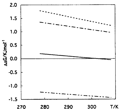
Figure 3. Temperature dependence of enantiomer selectivity for the complexation of ( S,R,R,S )- 2 with amines; 16 (- · · -), 17 (—), 18 (- · · ·), 19 (- - -).
